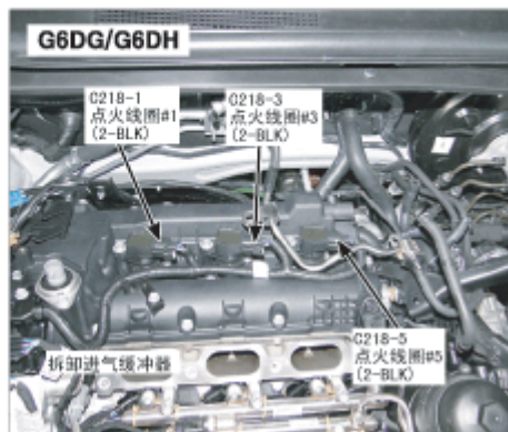
48. 发动机顶侧
