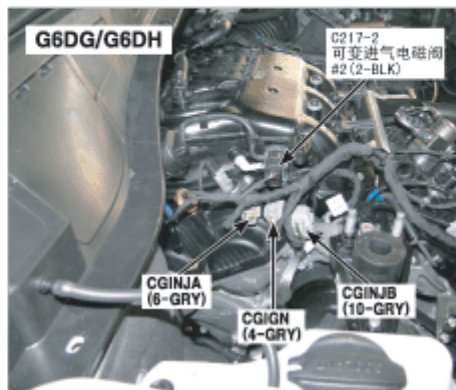
44. 发动机后右
