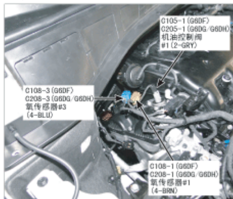
45. 发动机后右
